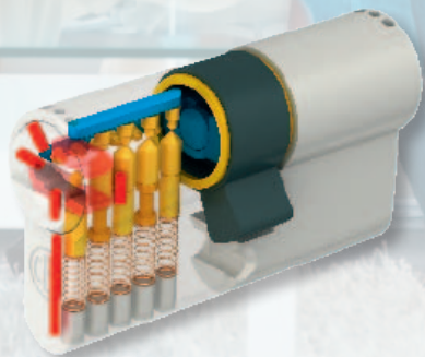
Sicherheits-Profilzylinder 910 WR
