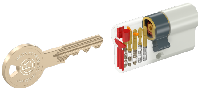
Abb.: 5-stiftiges System
