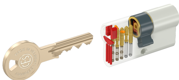
Fig.: Cylindre à 5-goupilles
